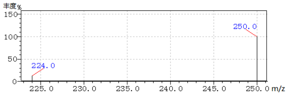
图 A.3 苯并(a)芘气相色谱-串联四级杆质谱-质谱图
