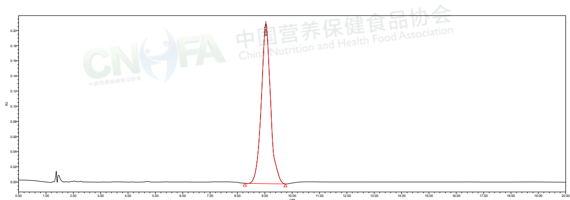
图 B.1 骨桥蛋白标准溶液 (0.5 mg/mL) 高效液相色谱图
