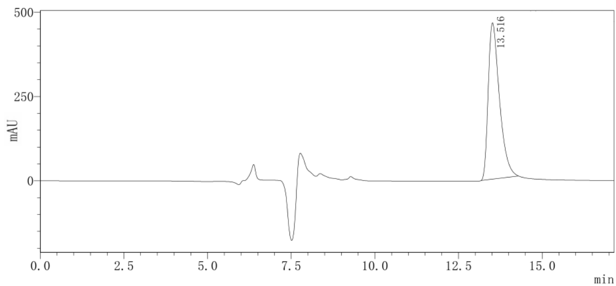
图B.1 硫酸胍基丁胺对照溶液高效液相色谱图
